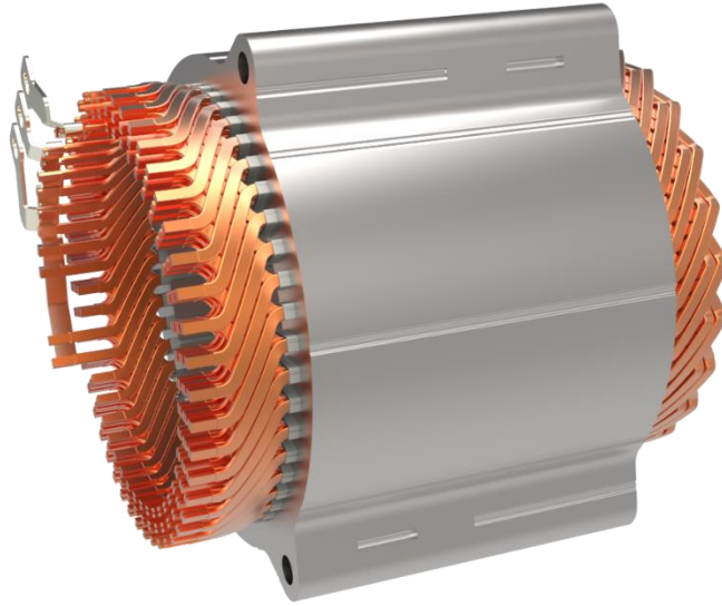
Tecnología de estator de horquilla de BorgWarner
