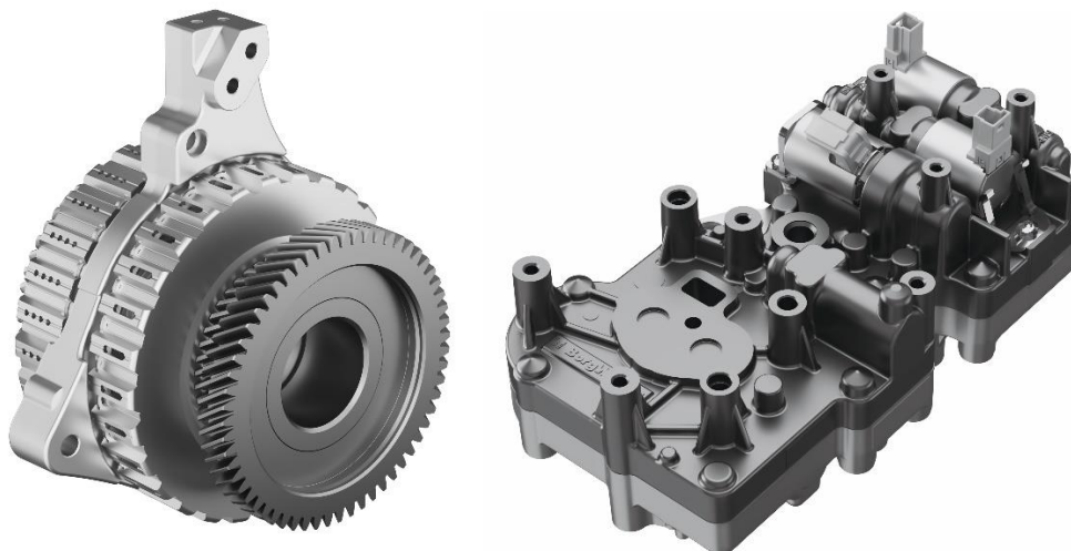
Embreagem úmida BorgWarner (esquerda) e módulo de controle hidráulico (direita)
