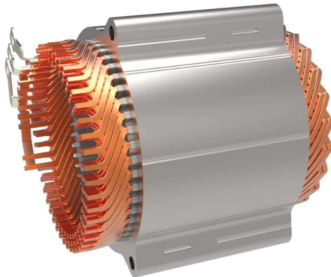
Die Hairpin-Statorwicklungstechnologie von BorgWarner
